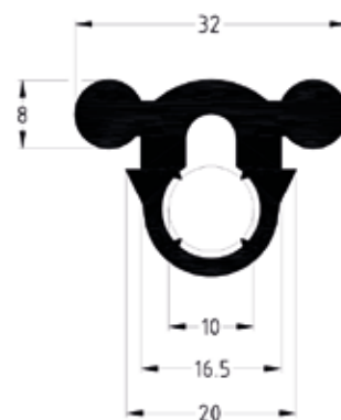
Für Profile 38/24 bis 40/120
