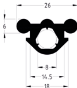
Für Profile 27/18 und 28/30
