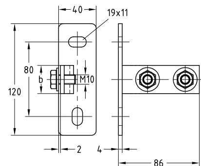
MPC-Stirnflansch, längs
